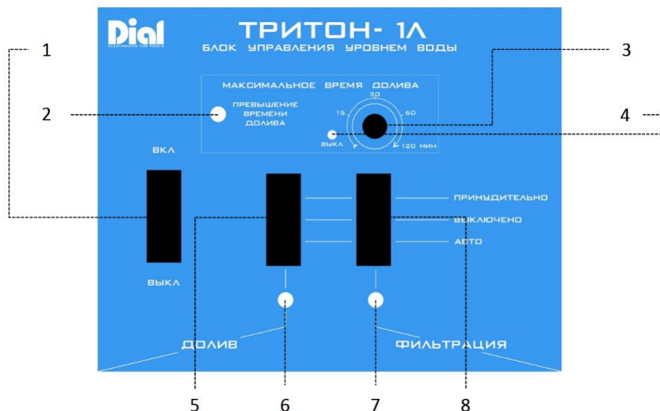
Рис. 1. Лицевая панель
