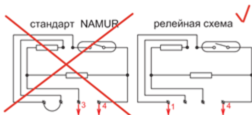
Рис. 4. Схема подключения счетчика VALTEC
