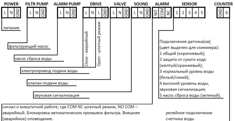
Рис. 3 Схема подключения
