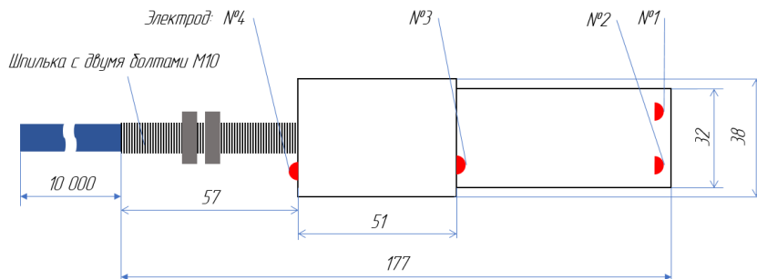
Рис. 5. Датчик уровня скиммерный трехуровневый ДС-2
