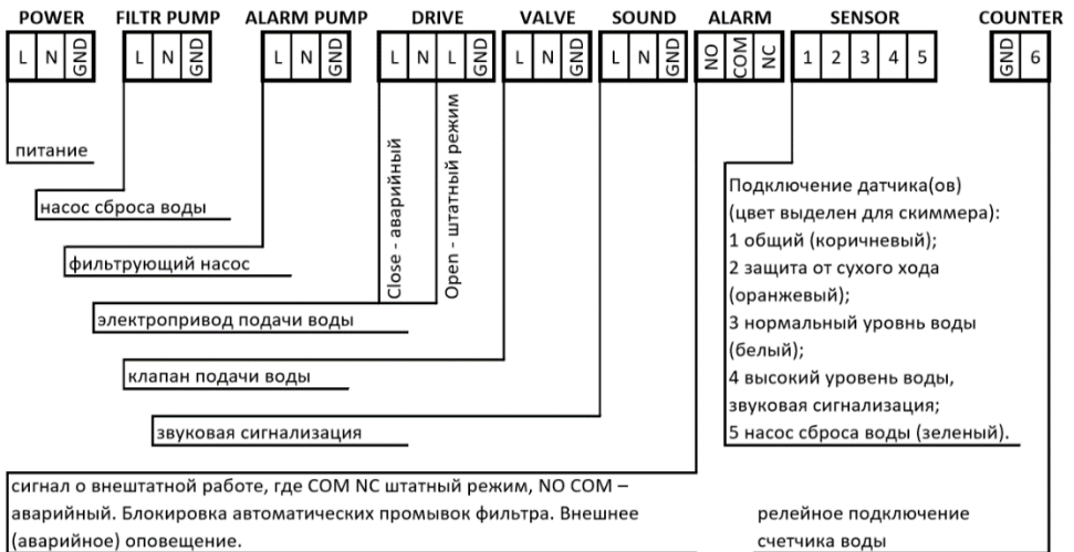
Рис. 3 Схема подключения
